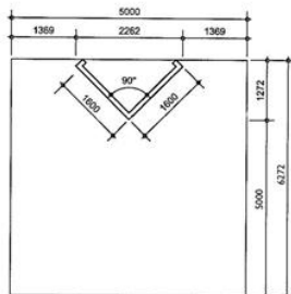
Oblique projection Schiefe Projektion
