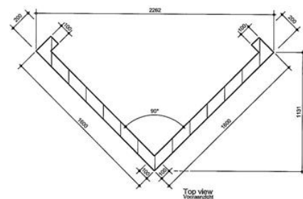
Top view Vorderansicht
